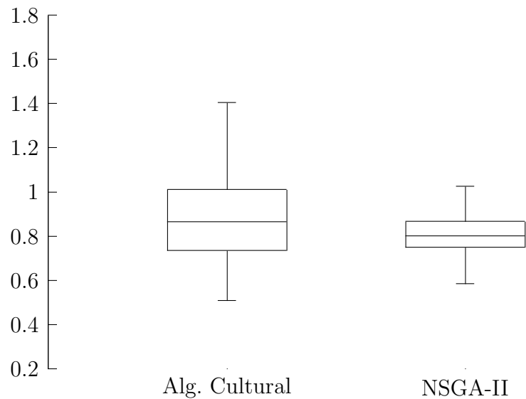
Figura D.15: Resultados del indicador de distribución en el problema ZDT6.
