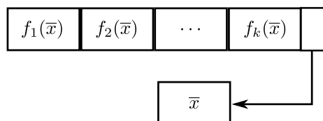
Figura 5.1: Cada punto en el espacio de creencias es un vector de valores de los objetivos. Además, cada punto incluye una referencia al vector de variables de decisión que lo generó.
