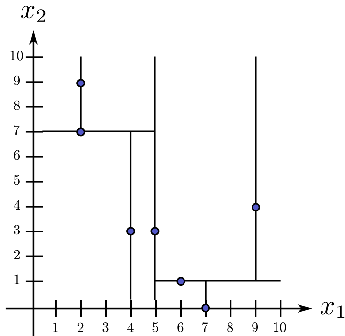
Figura 5.3: Partición del espacio determinada por el árbol del ejemplo 5.1.1.
